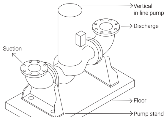
Installation type du support de pompe.
